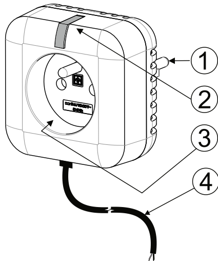
Fig. 1: 1 – fiche UniSchuko; 2 - bouton/indicateur de fonction ; 3 – prise française, 4 – câble de sortie commuté sans potentiel
